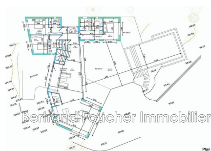
Plan RDC
